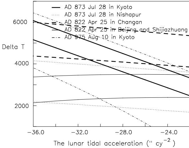
Fig. 4. (\Delta \dot{n}, \Delta T) 平面の皆既および金環食帯. 観測は, ほぼ同時代の紀元 873 年 7 月 28 日, 紀元 822 年 4 月 25 日, および 紀元 975 年 8 月 10 日の日食に関する 4 つの観測. 右に向かって上がる実線に囲まれた領域は, 紀元 822 年 4 月 25 日の日食の北京および石家荘の皆既帯を表す.
