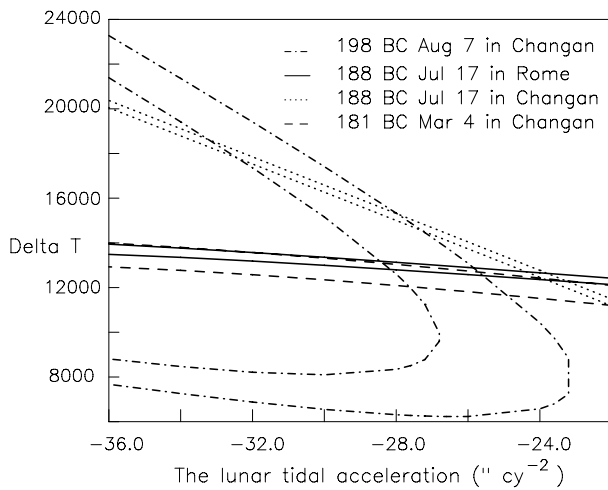
Fig. 2. 3つのほぼ同時代日食, 紀元前198年8月7日, 紀元前188年7月17日, and BC 181 Mar 4の4個の観測の (\Delta\dot{n}, \Delta T) 面の皆既または金環領域.
