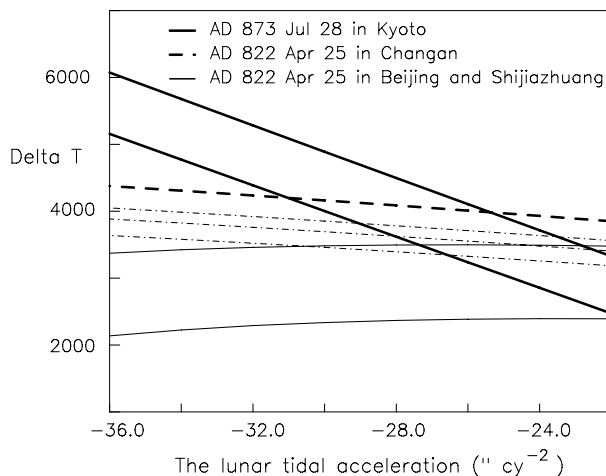
Fig. 5. ( \dot{n} , \Delta T ) における皆既食または金環食領域. 食はほぼ同時代の 紀元 873 年 7 月 28 日 および 紀元 822 年 4 月 25 日のものである. 点線は, 長安で観測された紀元 822 年 4 月 25 日の日食の皆既帯の下側境界を表す. 3 本のダッシュ線は, 紀元 822 年 4 月 25 日の日食を長安で観測したときの, 太陽円盤の残り角度が 90° (上), 105° (中), および 120° (下) となる軌跡を表す.
