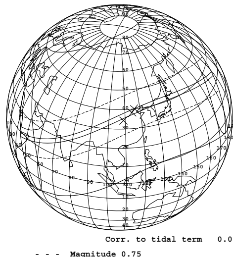
Fig. 6. 紀元 822 年 4 月 25 日の日食の皆既日食帯. ×印は南から長安, 石家荘, 北京を示す.
